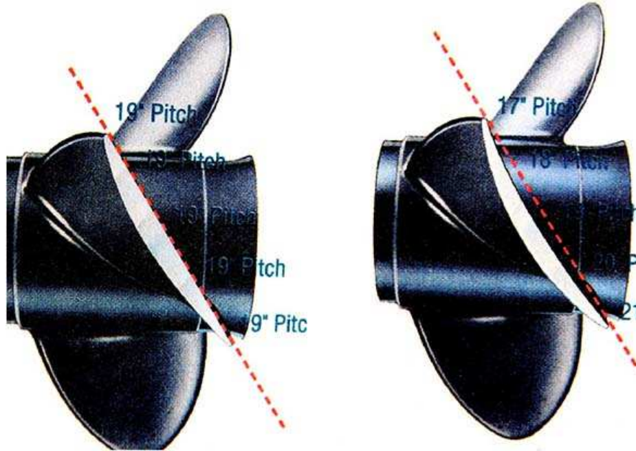
Έλικα με προοδευτικό βήμα
