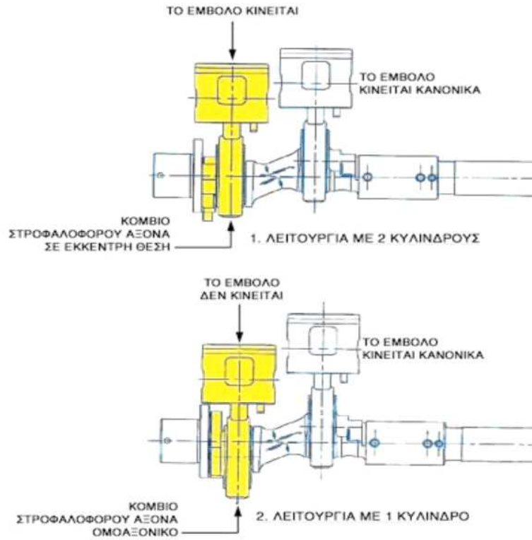
Στροφαλοφόρος άξονας και διωστήρας τύπου έκκεντρο
