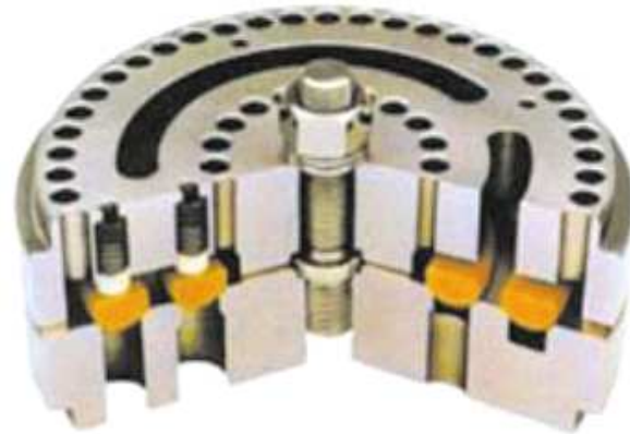
Τομή συγκροτήματος βαλβίδων δακτυλιοειδούς τύπου με την πλάκα βαλβίδων παλινδρομικών συμπιεστών
