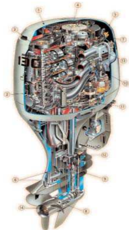
Τομή εξωλέμβιας μηχανής
