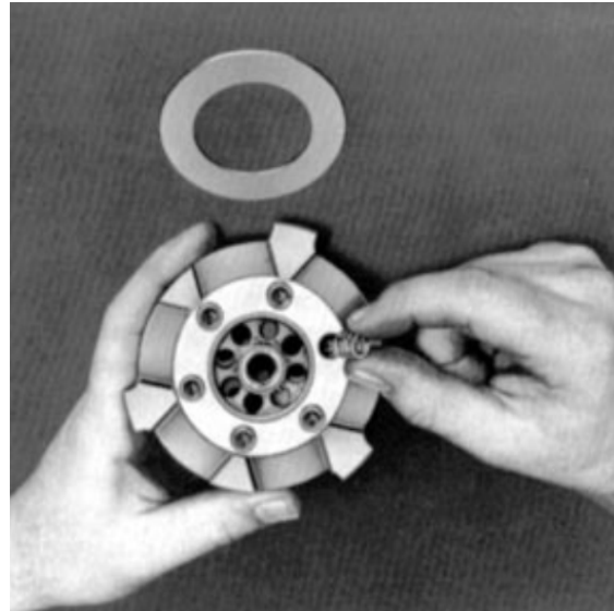
Δακτυλιοειδής βαλβίδα και πλάκα βαλβίδων με τα ελατήριά τους
