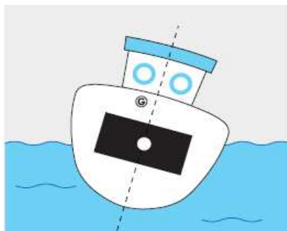
Πλήρης δεξαμενή: το κέντρο βάρους παραμένει σταθερό κατά την διατοίχιση του σκάφους
