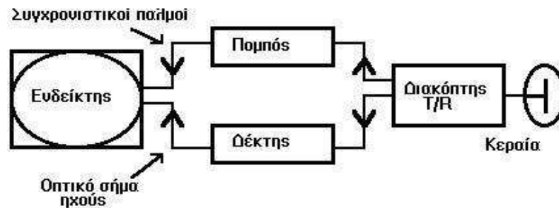
Σχεδιάγραμμα μερών και λειτουργίας του ραντάρ
