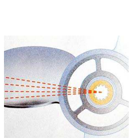
Το «κουπάρισμα» κατά μήκος της γραμμής του rake, μεταβάλλει το rake
