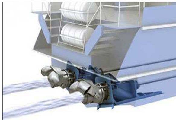
Water jet - Προωθητήρες αντίδρασης
