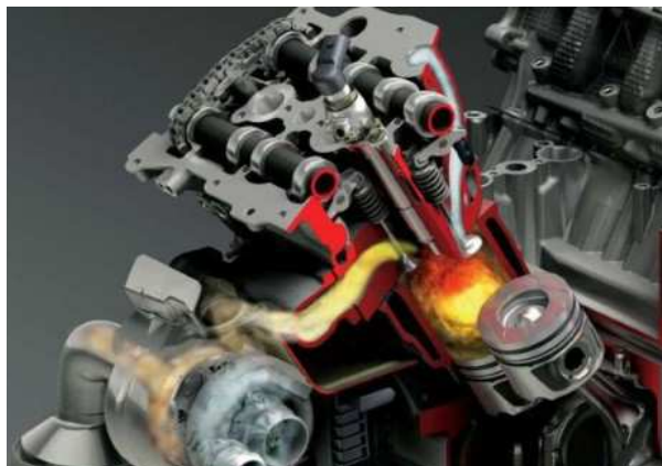
Θάλαμος καύσης κινητήρα DIESEL
