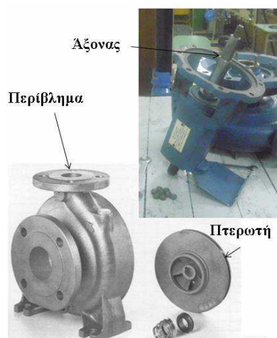
Φυγοκεντρική αντλία και τα κύρια μέρη της
