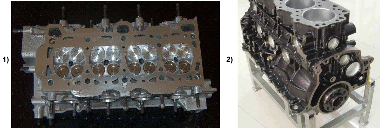
1) Κυλινδροκεφαλή με 4 βαλβίδες, δύο Εισαγωγής και δύο Εξαγωγής ανά κύλινδρο και 2) ο κορμός πετρελαιοκινητήρα
